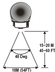
Montáž na pilíř nebo strom efektivní úhel
